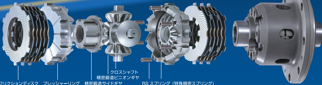
フリクションディスク プレッシャーリング 精密鍛造サイドギヤ クロスシャフト 精密鍛造ピニオンギヤ RSスプリング (特殊精密スプリング)
